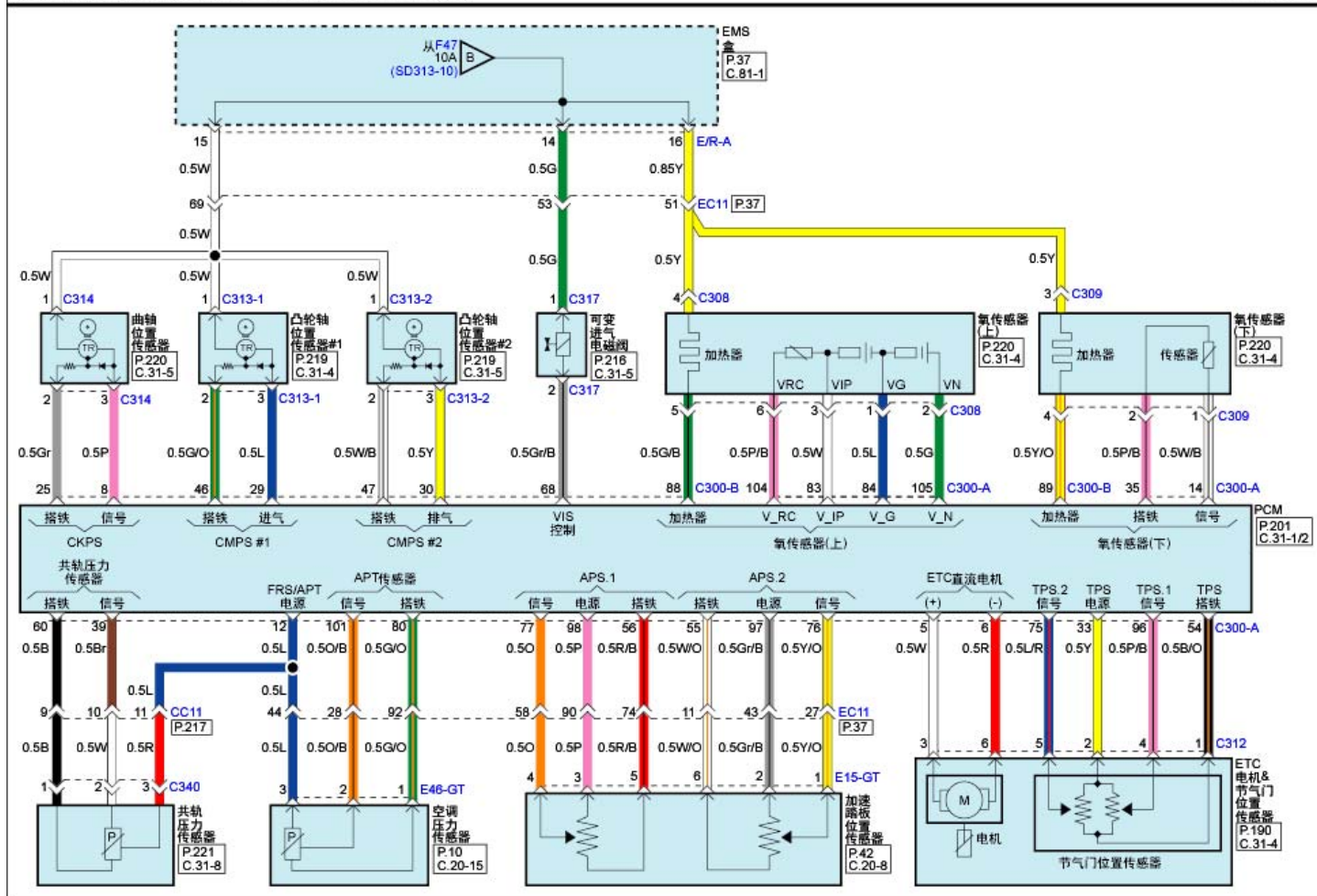
发动机控制系统(G4KJ : THETA-II 2.4L GDI)(4)
